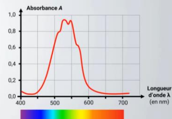
Spectre d'absorption d'une solution d'ions permanganate
